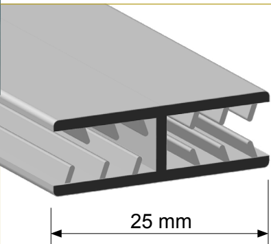
Ref. 4721 Perfil doble clipaje 180° Para espesores de 3 a 6 mm Material PVC / PVC Reciclado / Libre de PVC Ref. 4721 Double grip clip 180° 3 - 6 mm thickness materials PVC Material / PVC Free / Recycled PVC
