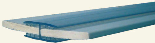
Ref. 4721 Perfil doble clipaje 180° Para espesores de 3 a 6 mm Material PVC / PVC Reciclado / Libre de PVC Ref. 4721 Double grip clip 180° 3 - 6 mm thickness materials PVC Material / PVC Free / Recycled PVC
